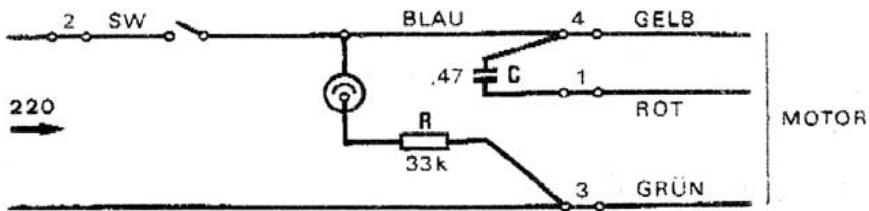
Fig. 3: Elektr. Schaltbild
